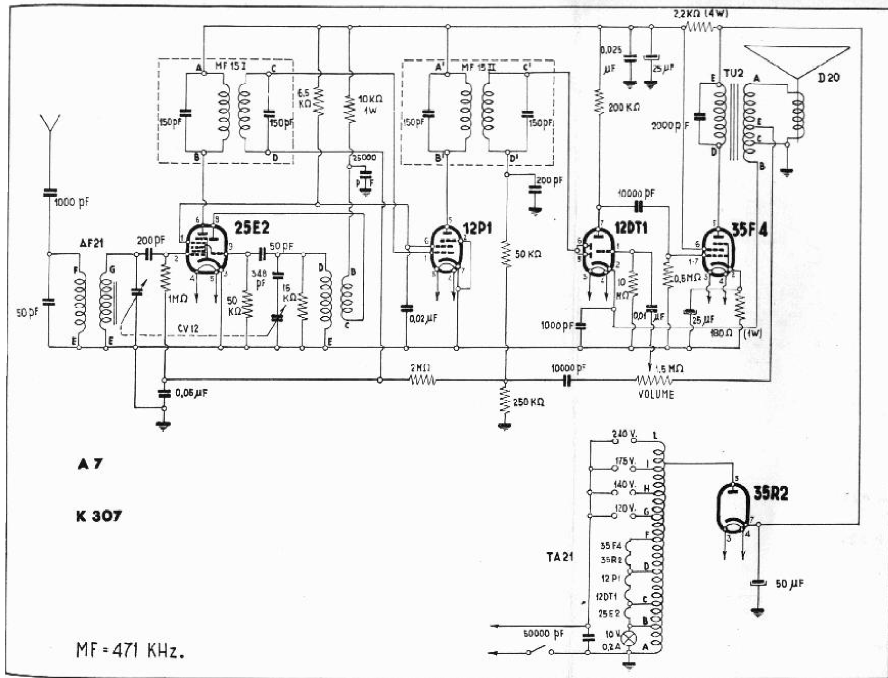
Modd. A 7 e K 307. Apparecchio AM per la gamma delle onde medie. Media frequenza a 471 kc/s. Potenza d'uscita 2 watt. Le valvole portano la numerazione Magnadyne.
